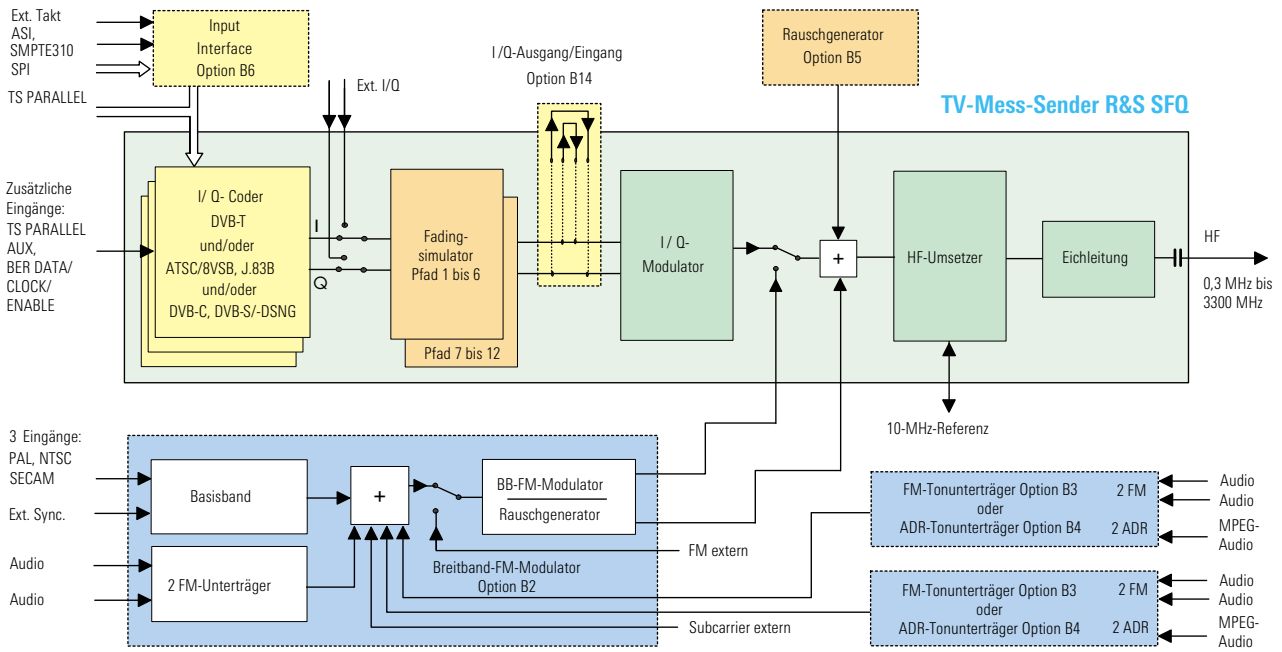
Prinzipialschaltung des TV-Messsenders R&S SFQ mit den möglichen Optionen
